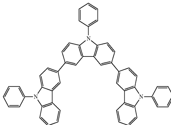
Tris-PCz
