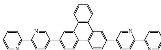
BPt-TP2
